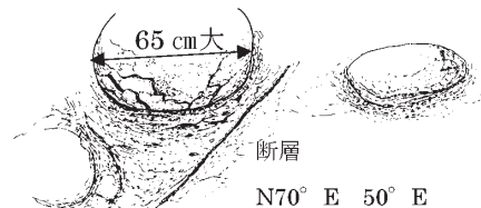
図5 散在する球状風化と断層
