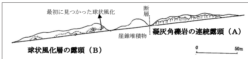
図4 断層亀裂の多い凝灰角礫岩の露頭 (A)
