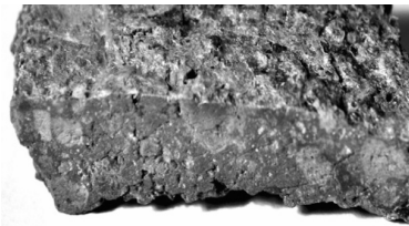
Ph19 拡大 落下した風化殻の破片
