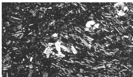
Ph2 クロスニコル
