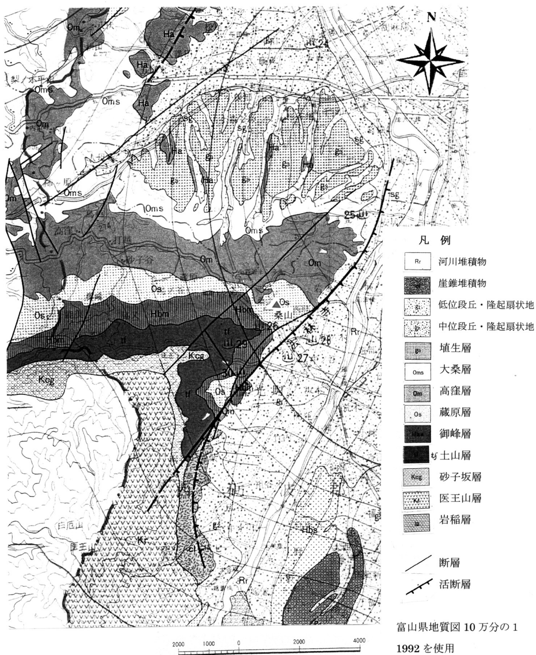
図1 桑山周辺の地質図
