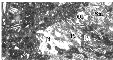
Ph1 シングルニコル
