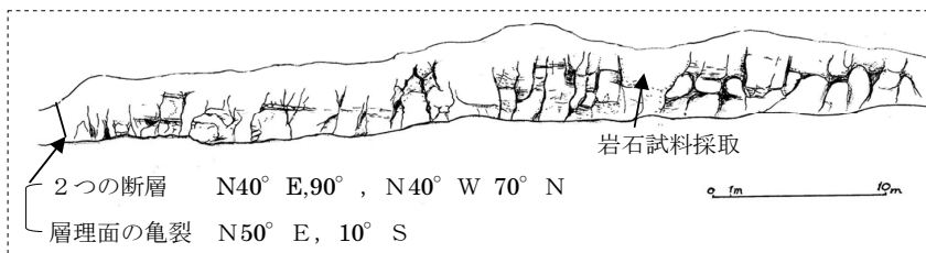
図4 断層亀裂の多い凝灰角礫岩の露頭 (A)
