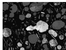
Ph8 クロスニコル
