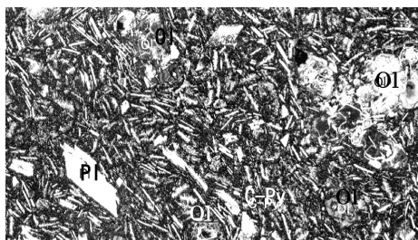
Ph5 シングルニコル
