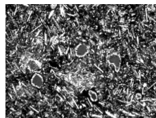
Ph10 クロスニコル
