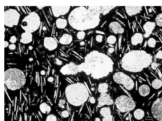
Ph7 シングルニコル
