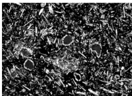
Ph21 桑山石採掘場跡の角礫
