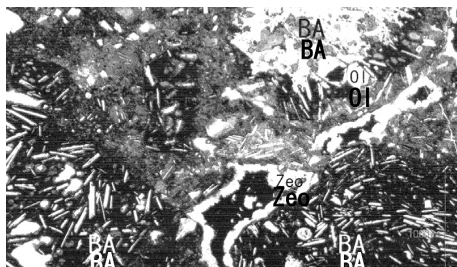
Ph3 シングルニコル
