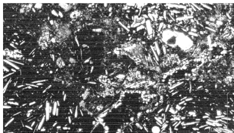
Ph4 クロスニコル
