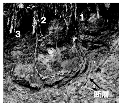
Ph16 落下跡の風化殻と痕跡の露出
