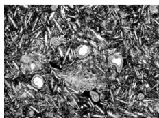
Ph9 シングルニコル
